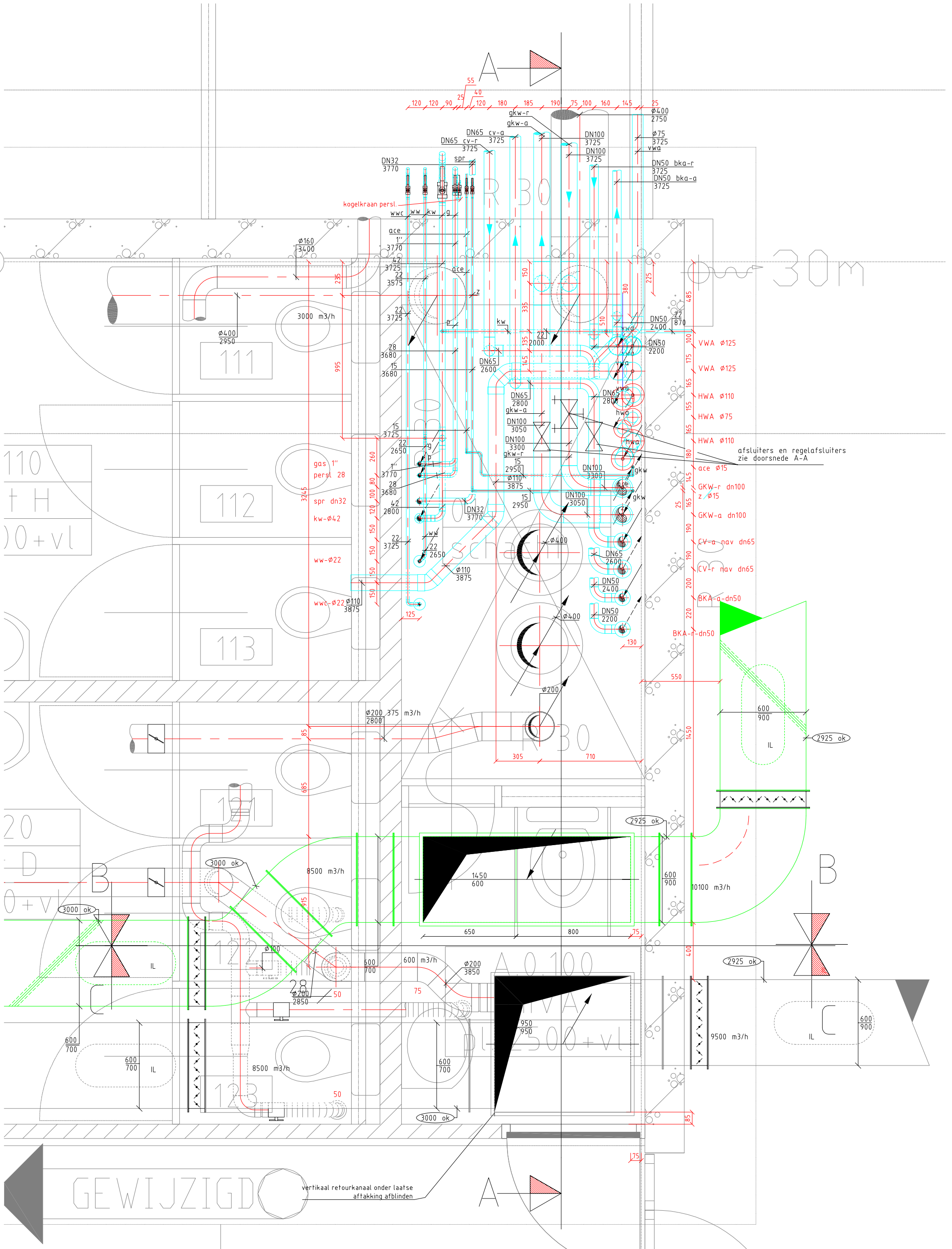
PLATTEGROND BG PLAFOND
